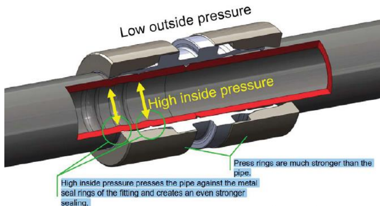
Funktionsweise Haelok-Verbindungstechnik
